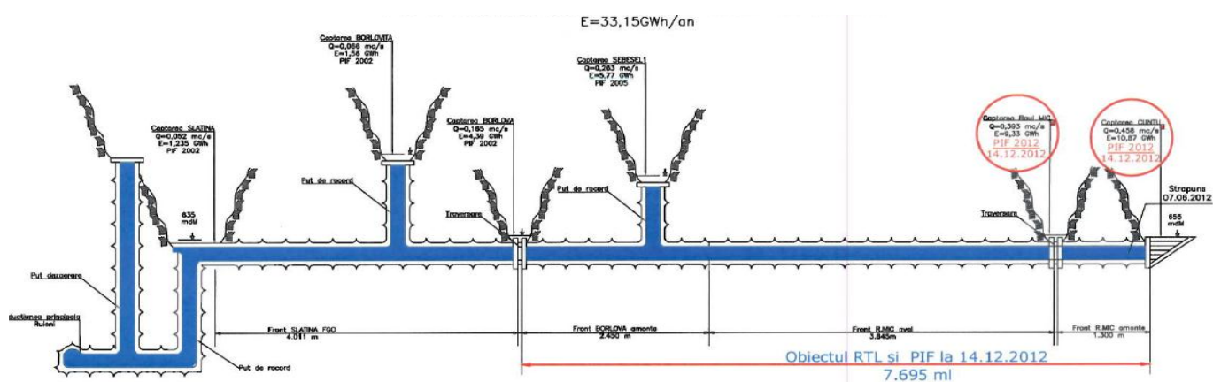
Aducțiunea secundara Sebes-Ruieni. Tronson receptionat la 14.12.2012
